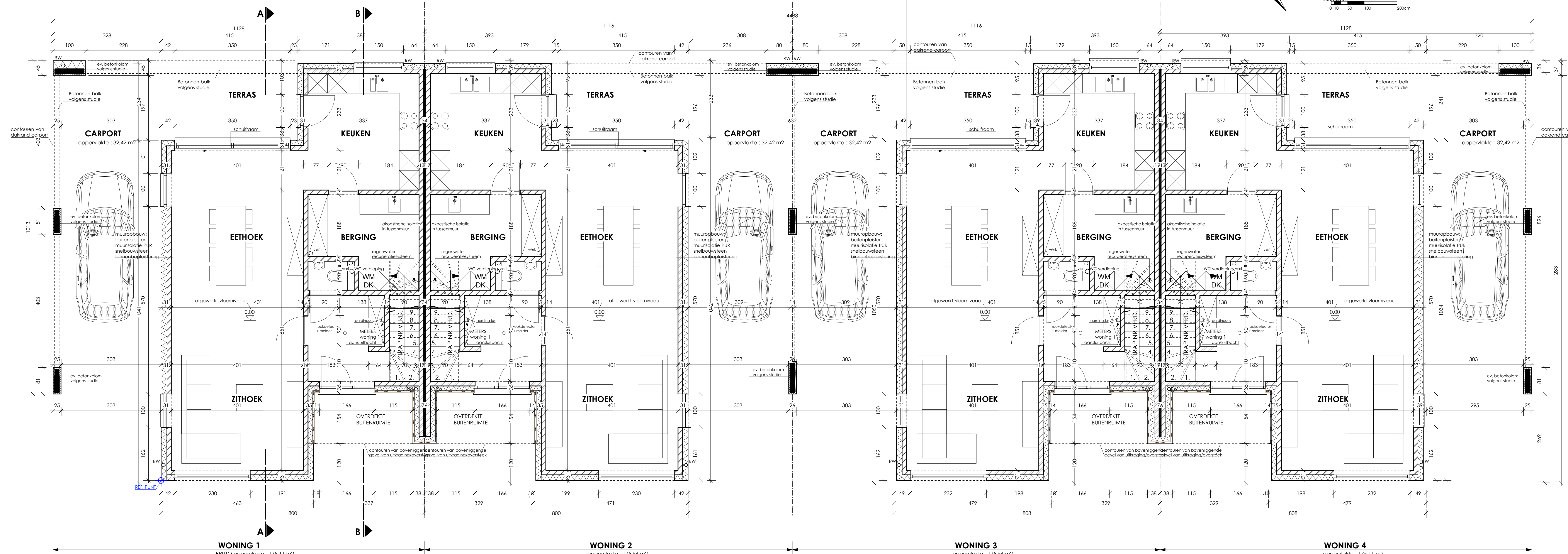
GRONDPLAN
